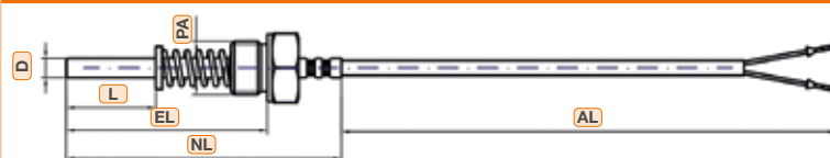
Kabelfühler mit loser Verschraubung Außengewinde, Druckfeder Schutzhülse verjüngt
