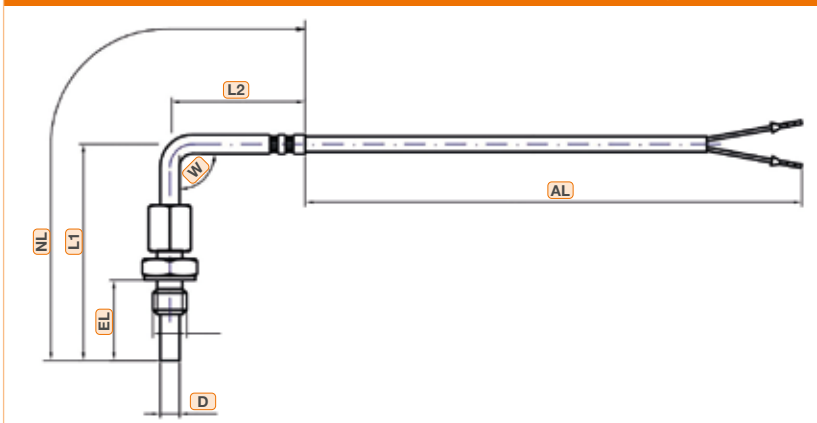
Kabelfühler mit gebogener Schutzhülse, mit Klemmverschraubung
