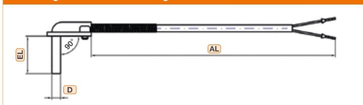
Mehrteiliges Schutzrohr 90° abgewinkelt
