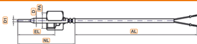
Kabelfühler mit Verschraubung (fest) Innengewinde, Schutzhülse verjüngt
