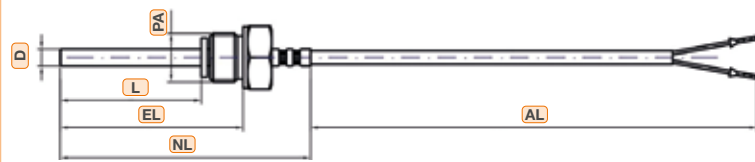
Kabelfühler mit loser Verschraubung, Außengewinde, Schutzhülse verjüngt
