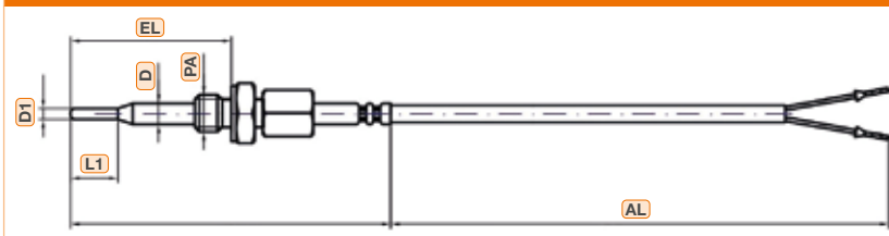
Kabelfühler mit verjüngter Schutzhülse, mit Klemmverschraubung
