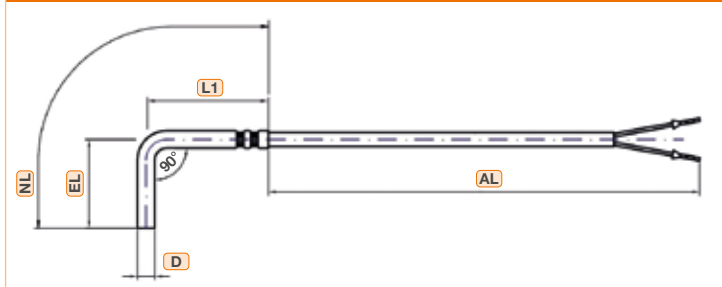
Schutzhülse gebogen
