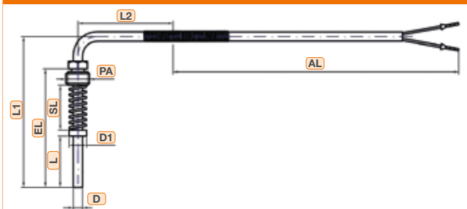
Kabelfühler gewinkelt, mehrteiliger Schraubverbinder, lose Verschraubung, mit Druckfeder
