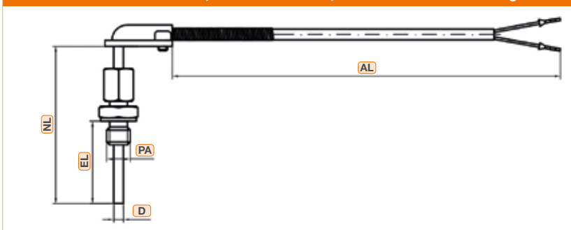
Kabelfühler mit Schutzhülse, Winkelanschluss, mit Klemmverschraubung
