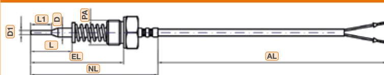
Kabelfühler mit loser Verschraubung, Innengewinde, Druckfeder
