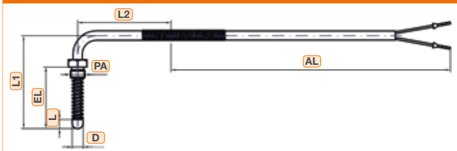
Kabelfühler gewinkelt, lose Verschraubung mit Druckfeder
