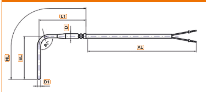
Schutzhülse gebogen und verjüngt
