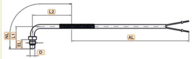
Kabelfühler gewinkelt, mehrteiliger Schraubverbinder, lose Verschraubung
