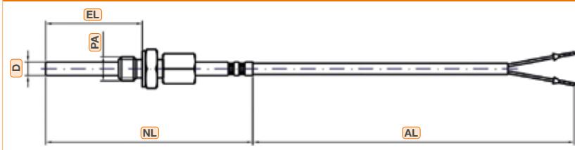
Kabelfühler mit metallischer Schutzhülse, mit Klemmverschraubung
