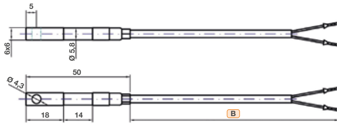
Kabelfühler mit Universal Anschraubklotz mit Befestigungsloch und für Spannbandmontage (Konstruktion 1)
