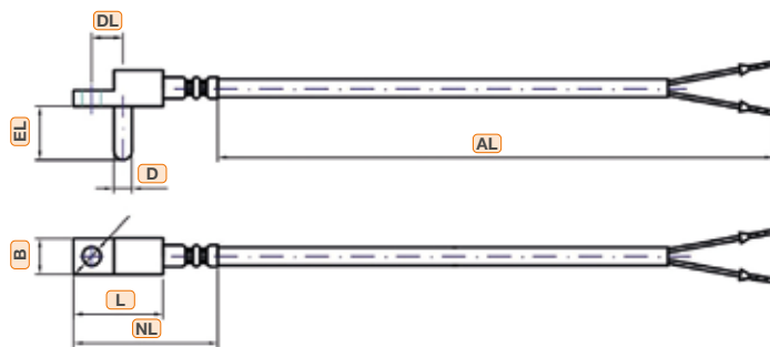
Kabelfühler mit Anschraubklotz mit Stift und Befestigungsloch (Konstruktion 4)
