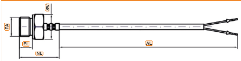
Kabelfühler Schutzhülse mit Gewinde mit Sechskant
