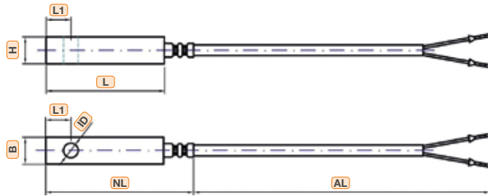
Kabelfühler mit Anschraubklotz und Befestigungsloch (Konstruktion 2)
